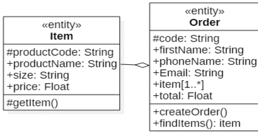
Рисунок 3.28 – Агрегація між класами Товар ( Order ) і Замовлення ( Item )
