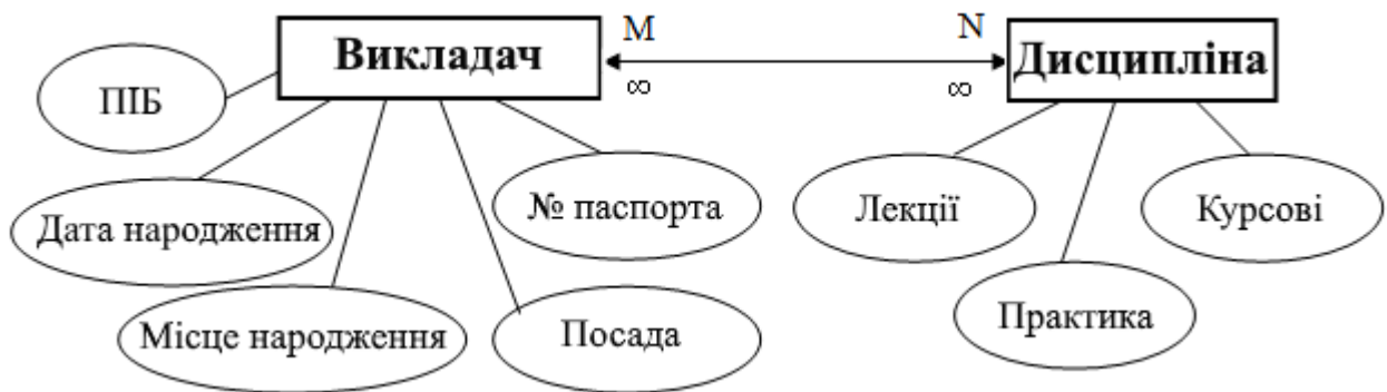
Рисунок 3.79 – Інфологічна модель Викладач-Дисципліна
