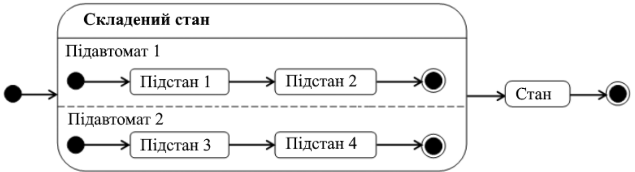
Рисунок 3.71 – Приклад стану з непорожньою секцією внутрішніх дій
