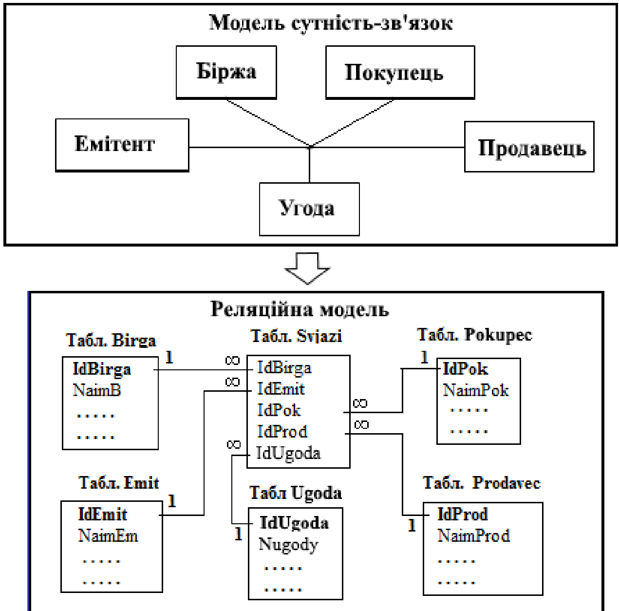
Рисунок 3.86 – Перетворення моделі сутність-зв'язок зі зв'язком степені K у реляційну модель
