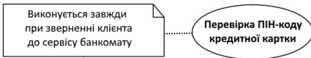
Рисунок 3.8 – Приклад коментарів у мові UML
