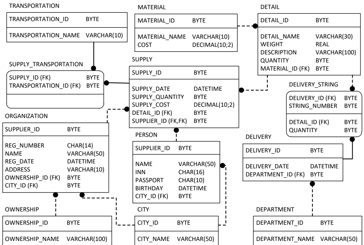
Рисунок 3.91 – Фізична модель бази даних: реалізація наслідування через міграцію предка в нащадків
