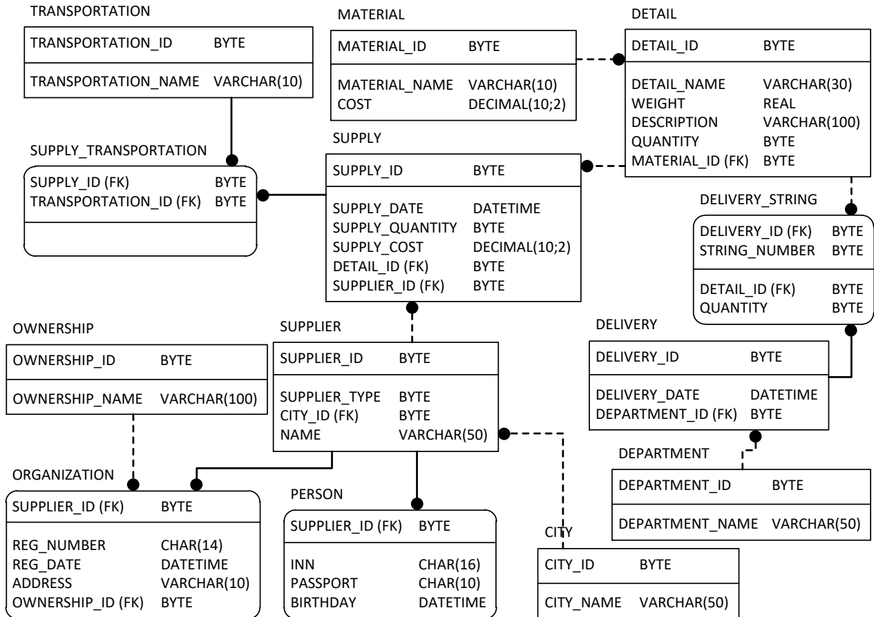
Рисунок 3.92 – Фізична модель бази даних: реалізація наслідування через заміну ієрархії ідентифікуючими зв'язками
