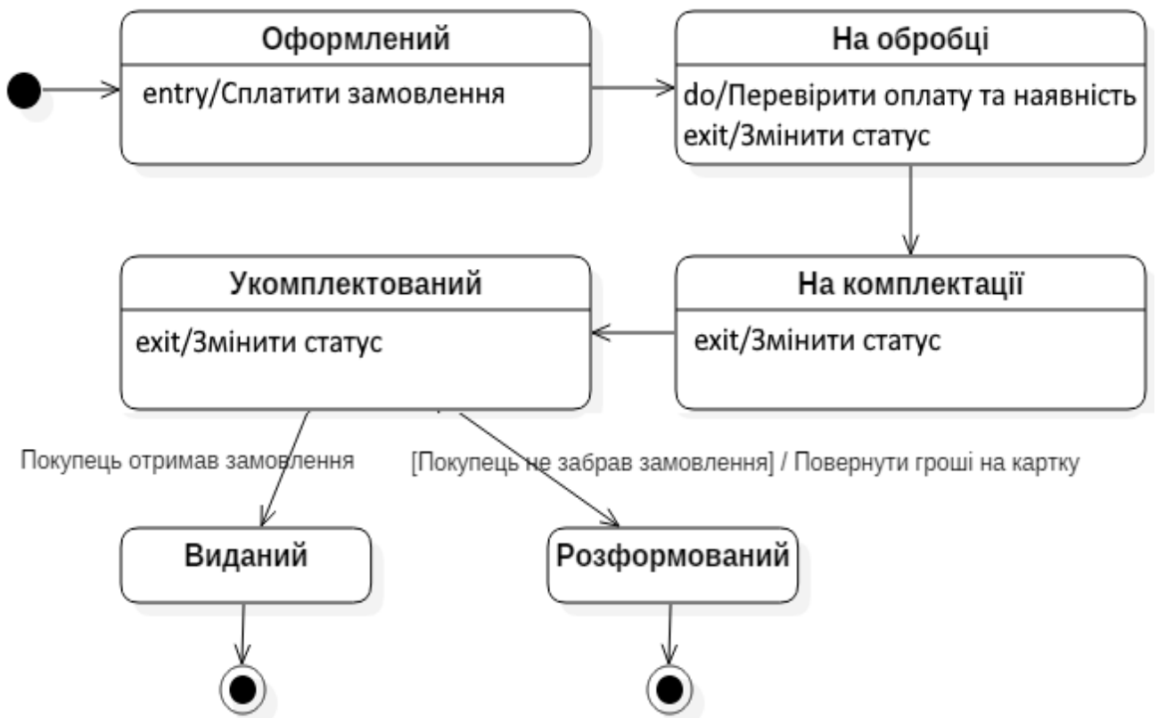
Рисунок 3.75 – Остаточна діаграма станів об'єкту Замовлення
