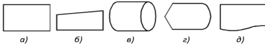
Рисунок 4.1 – Основні графічні символи для опису функціональної схеми ПЗ: а) – процес, підсистема; б) – ручне введення; в) – пристрій пам'яті з прямим доступом; г) – дисплей; д) – документ
