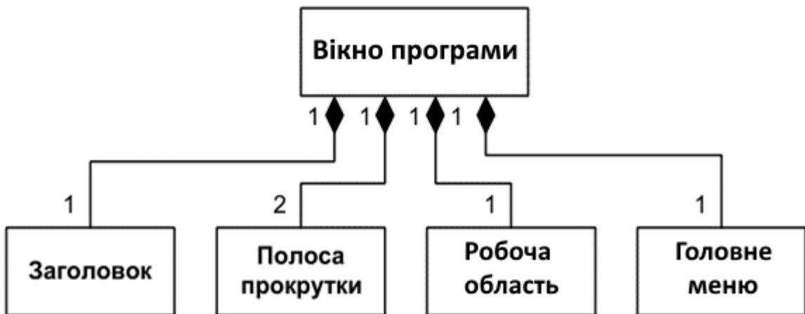
Рисунок 3.30 – Діаграма класів для ілюстрації відношення композиції
