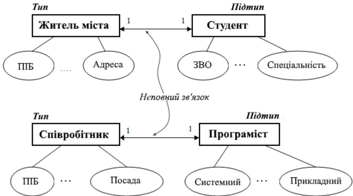
Рисунок 3.81 – Тип і підтип сутностей
