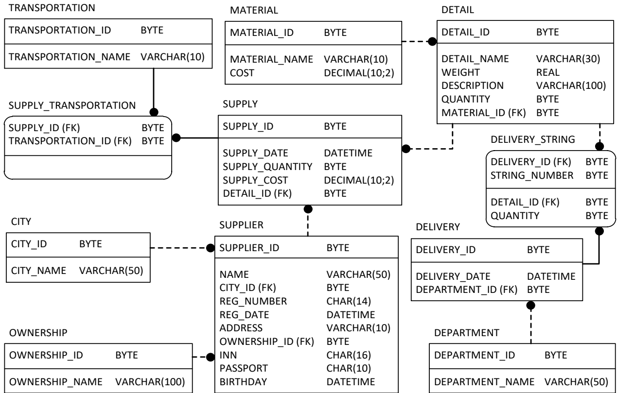
Рисунок 3.90 – Фізична модель бази даних: реалізація наслідування через міграцію нащадків у предка
