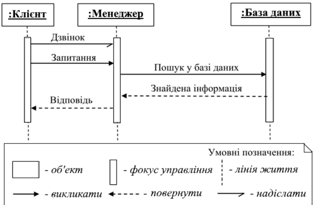
Рисунок 3.64. Фрагмент діаграми послідовності
