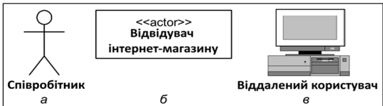
Рисунок 3.7 – Варіанти символів графічного позначення актора: а – у вигляді «дротяного чоловічка»; б – у вигляді прямокутника; в – у формі піктограми
