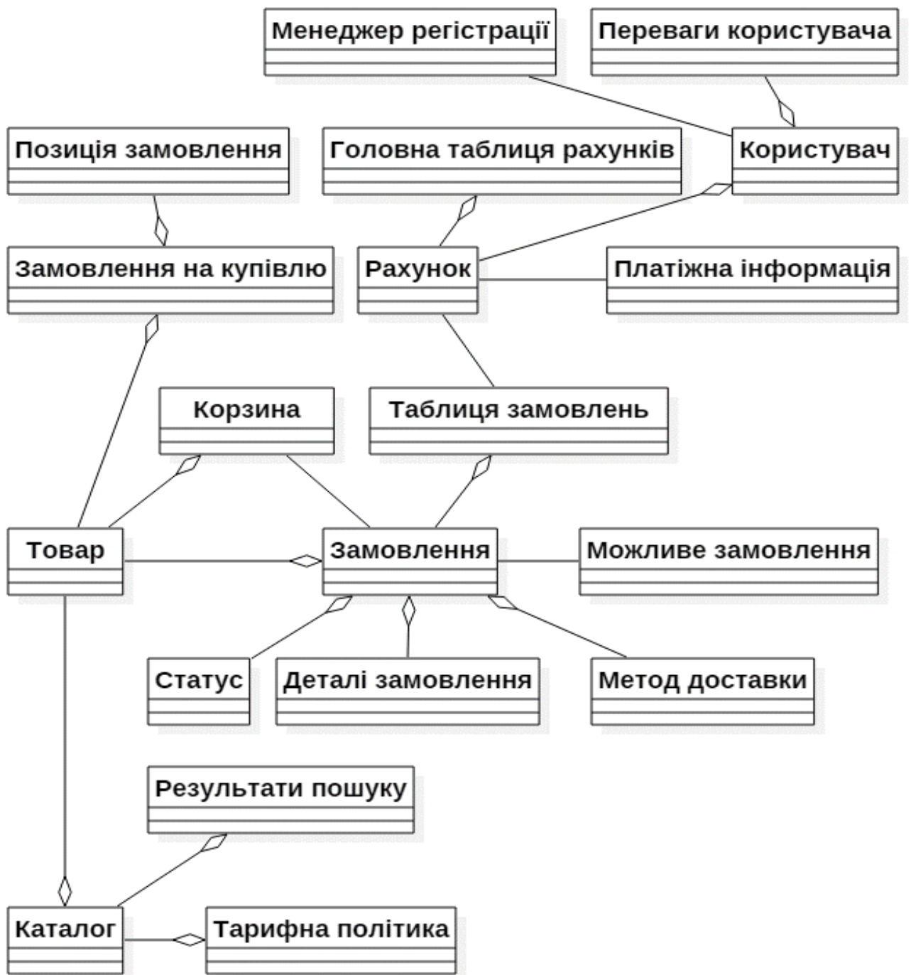
Рисунок 3.5 – Модель предметної області internet-магазину
