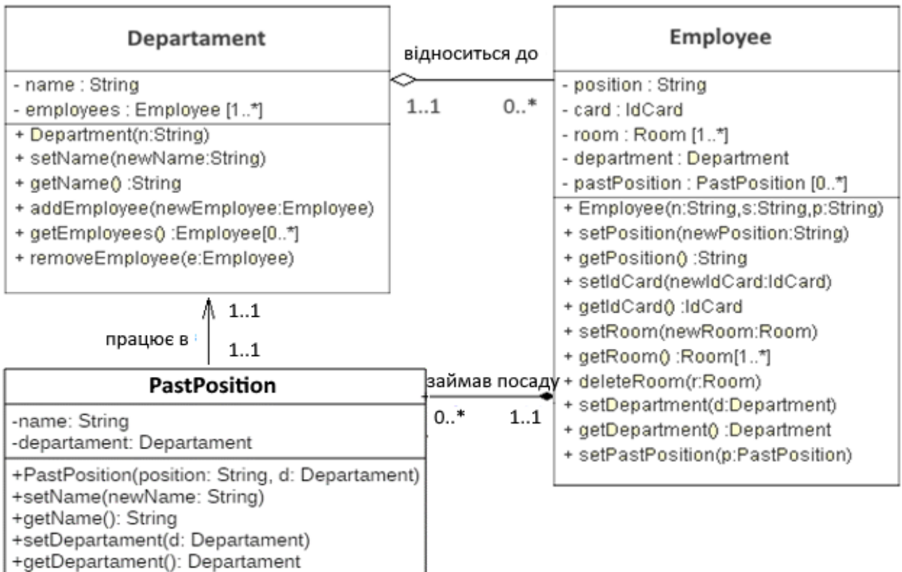
Рисунок 3.40 – Відношення композиції
