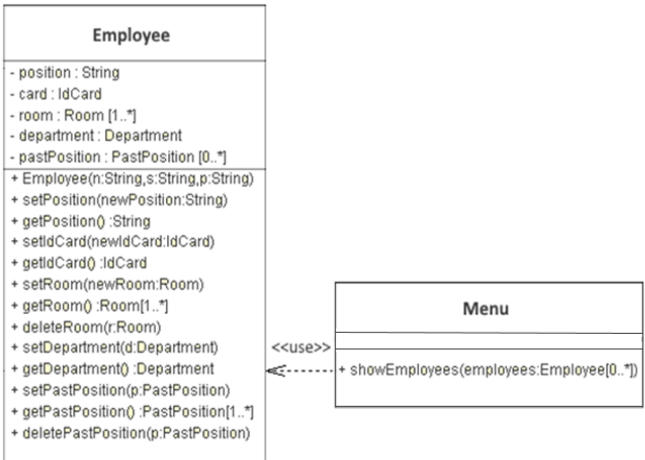
Рисунок 3.41 – Відношення залежності
