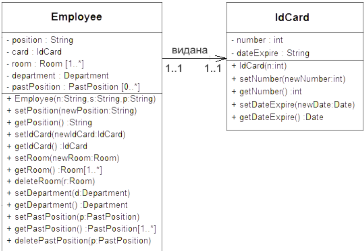
Рисунок 3.37 – Бінарна асоціація
