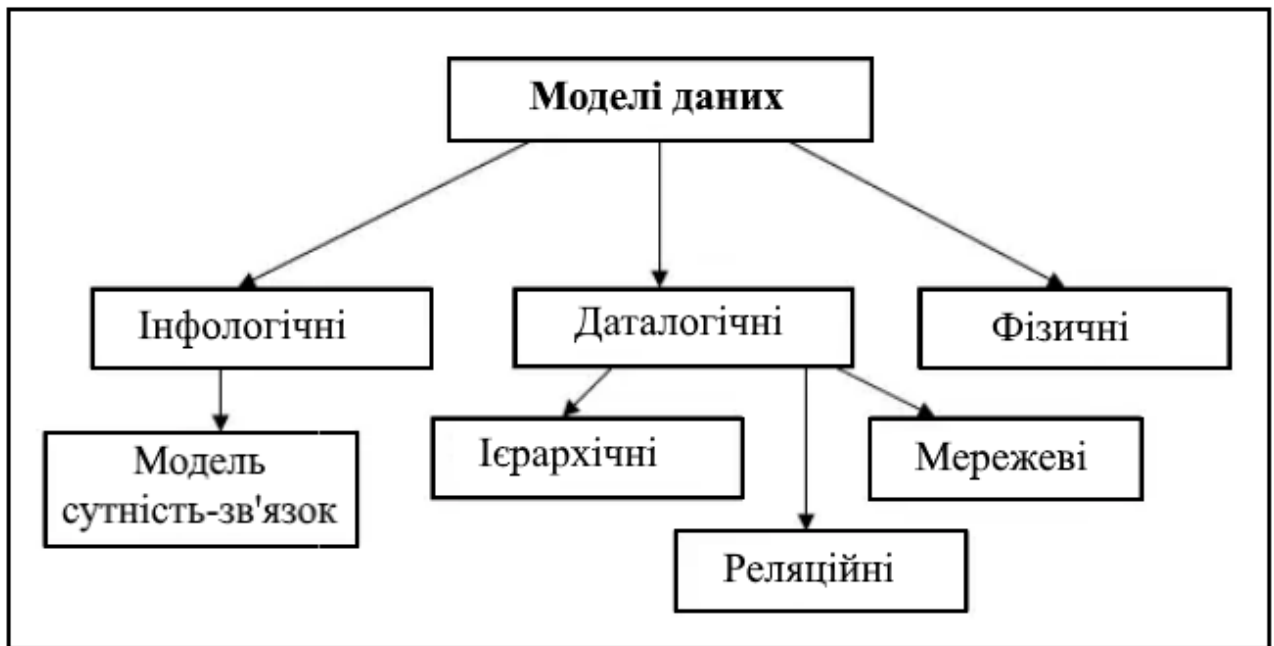
Рисунок 3.77 – Моделі даних
